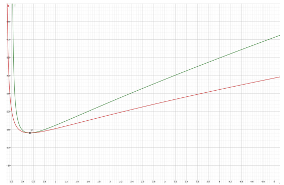
Curva di Paschen classica / corretta dello Xeno
